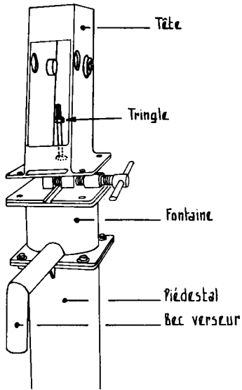
Montage de la tête de la pompe India
